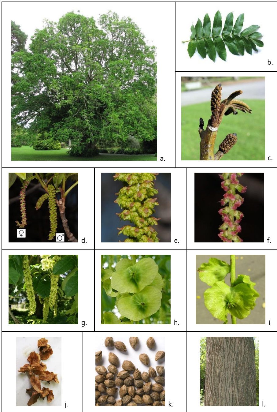
Noce del Caucaso - a) pianta adulta; b) foglia; c) fase di germogliamento; d) infiorescenze maschile e femminile; e) fiori maschili; f) fiori femminili; g) infruttescenze; h-i) frutti in fase di sviluppo; j) frutti maturi; k) semi; l) corteccia di pianta adulta.
