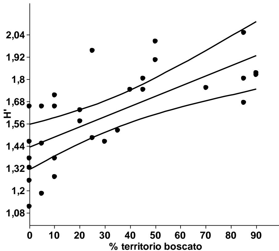
Fig. 1: correlazione bosco/biodiversità (H') su 30 siti dell'Italia centrale tirrenico-collinare; ambito di confidenza = 95%; correlazione: r > 0,69 ; Spearman: p < 0,01 ; Kendall: p < 0,01 ; software "PAST".
