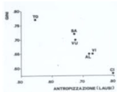
Fig. 2: antropizzazione (Lausi, modif.) / biodiversità (Gini) nei distretti vulcanici dell'alto Lazio.
